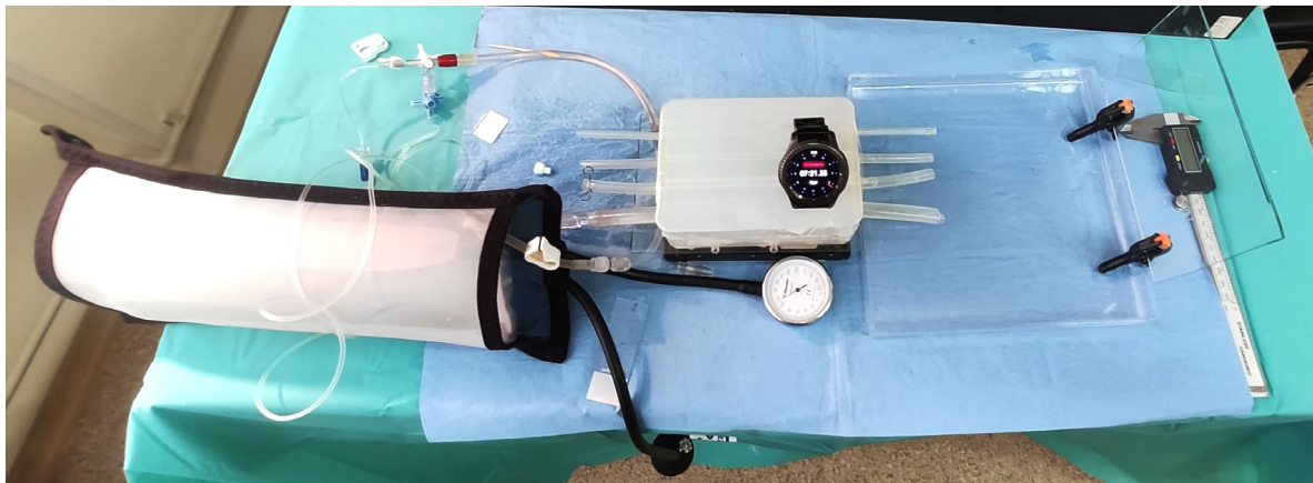
Рисунок 5. Стенд для испытания сопротивления обтурирующего конгломерата из геля «LeGoо» и созданного композита напору жидкости
